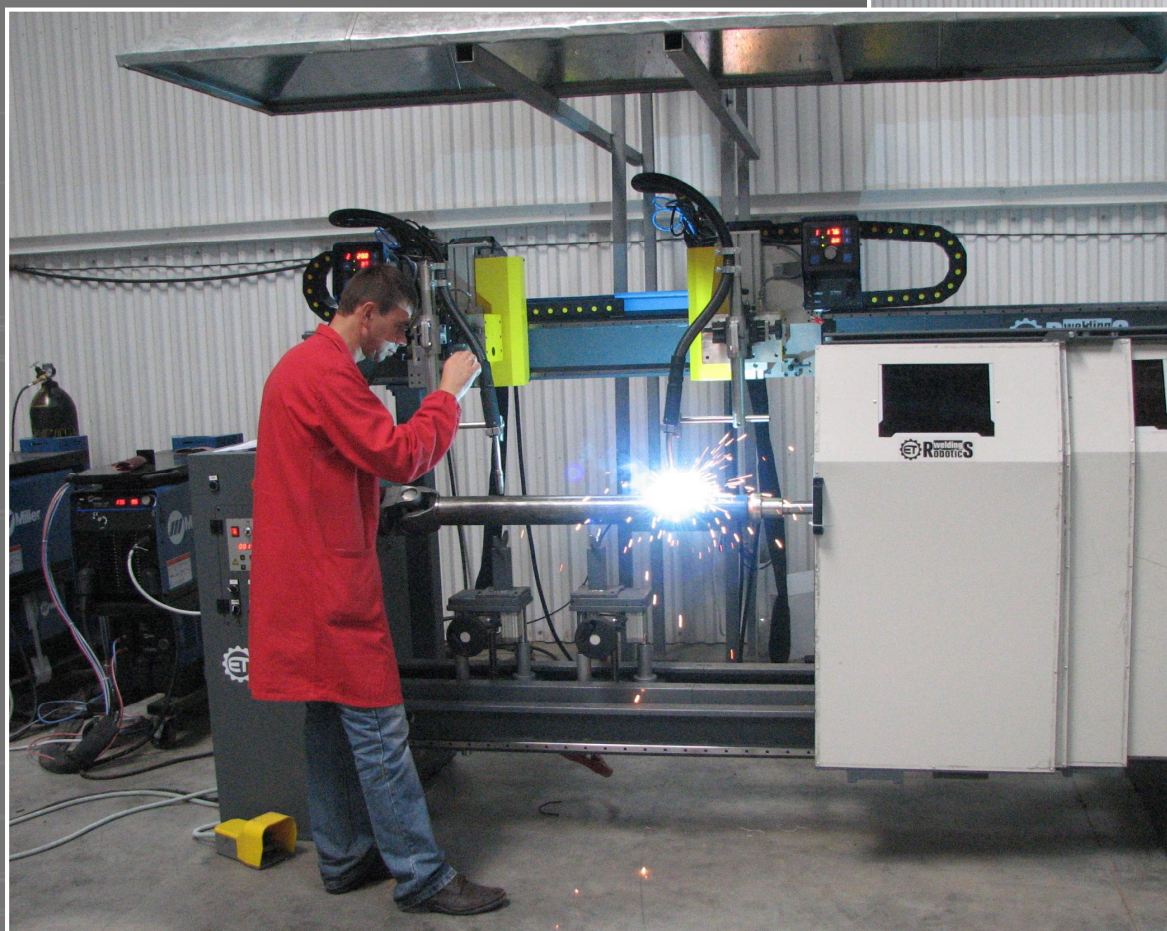
Машина для автоматической MIG сварки двух кольцевых швов
